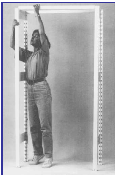
Az állványkeretet alul és felül hossztartóval kapcsolja össze!
